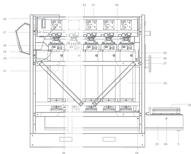
VISTA LATERALE DESTRA
